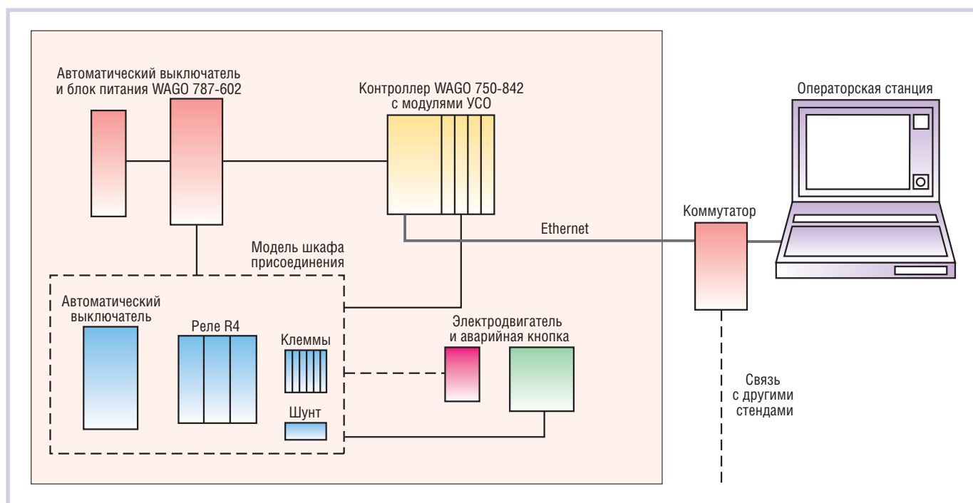
Рис. 2. Структура лабораторного стенда
